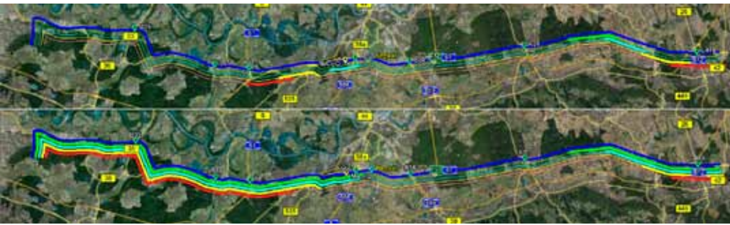
Ablaufsimulation im Satellitenbild: Das obere Bild zeigt in der KW 37 den Bereich, in dem die jeweiligen Kolonnen farblich gekennzeichnet aufeinanderfolgend arbeiten, das untere alle Arbeiten, die bis zur KW 37 erledigt sind
